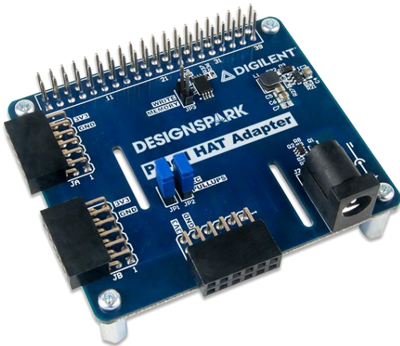
The Pmod HAT Adapter
